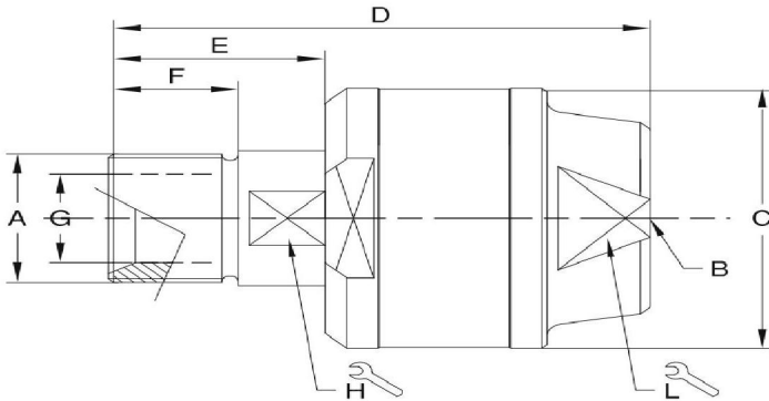
M G0450高速旋转接头尺寸图
