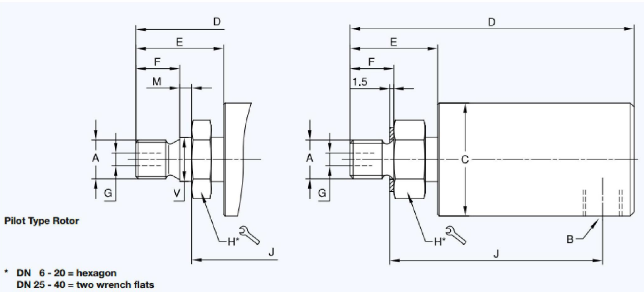
M G035高速旋转接头尺寸图
